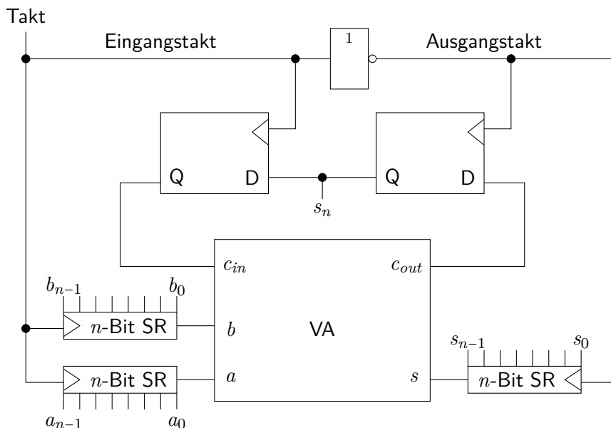
Abbildung 4.6: Serielladdierer
