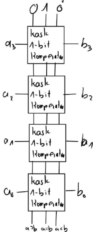
Abbildung 5.7: kaskadierbarer 4-Bit-Komparator
